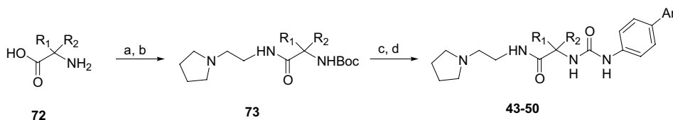
Scheme 4. Reagents: (a) (\text{BOC})_2\text{O} , \text{Me}_4\text{NOH}\cdot\text{H}_2\text{O} , \text{CH}_3\text{CN} ; (b) 2-ethylpyrrolidine amine, EDCI, HOBT, DMF, NMM; (c) 4 M HCl/dioxane, \text{CH}_2\text{Cl}_2 ; (d) \text{ArPhNCO} , \text{Et}_3\text{N} , \text{CH}_2\text{Cl}_2 .
