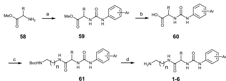
Scheme 1. Reagents: (a) ArNCO, Et 3 N, toluene; (b) LiOH, THF–H 2 O (3:1, v/v); (c) EDCl, HOBT, DMF, BocNH–(CH 2 ) n –NH 2 ; (d) CF 3 CO 2 H, CH 2 Cl 2 .
